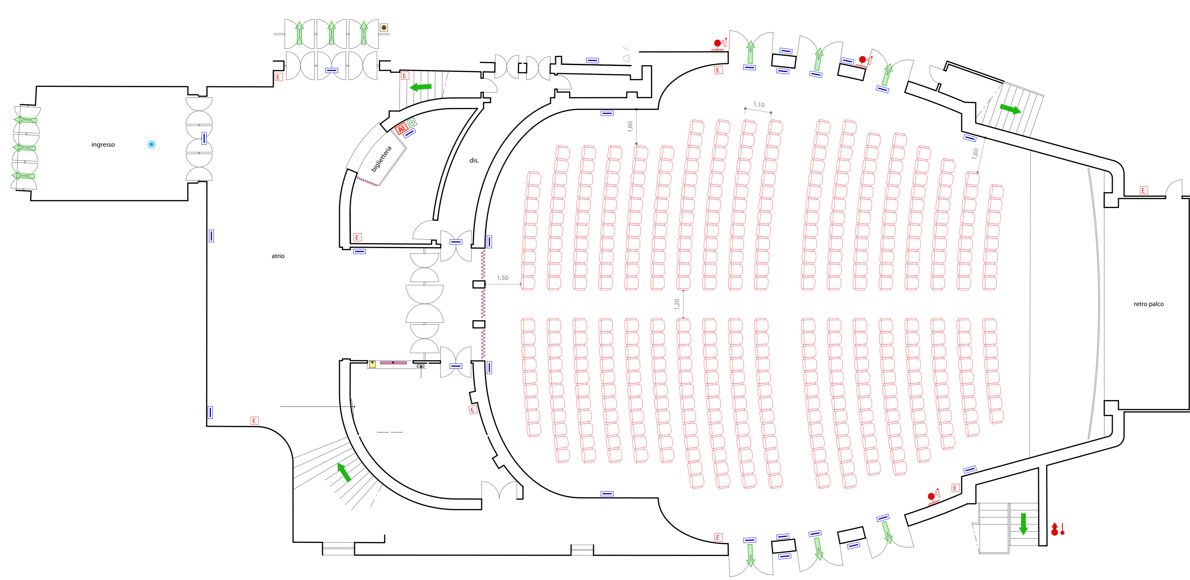
pianta platea scala 1/100
